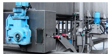
Lubrificação do rolamento da roda no raspador circular
